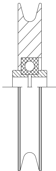
Ruote per porte basculanti
